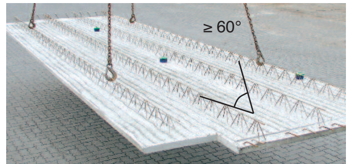
Bild 6: Winkel zwischen Gehänge und Deckenelement \geq 60^\circ
