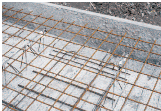
Bild 10: Obere Bewehrung und Fugenstoßbewehrung
